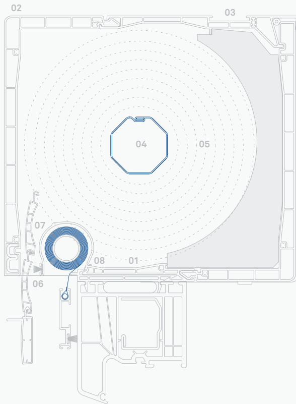
PROtex Rollladenaufsetzelement mit Insektenschutz
